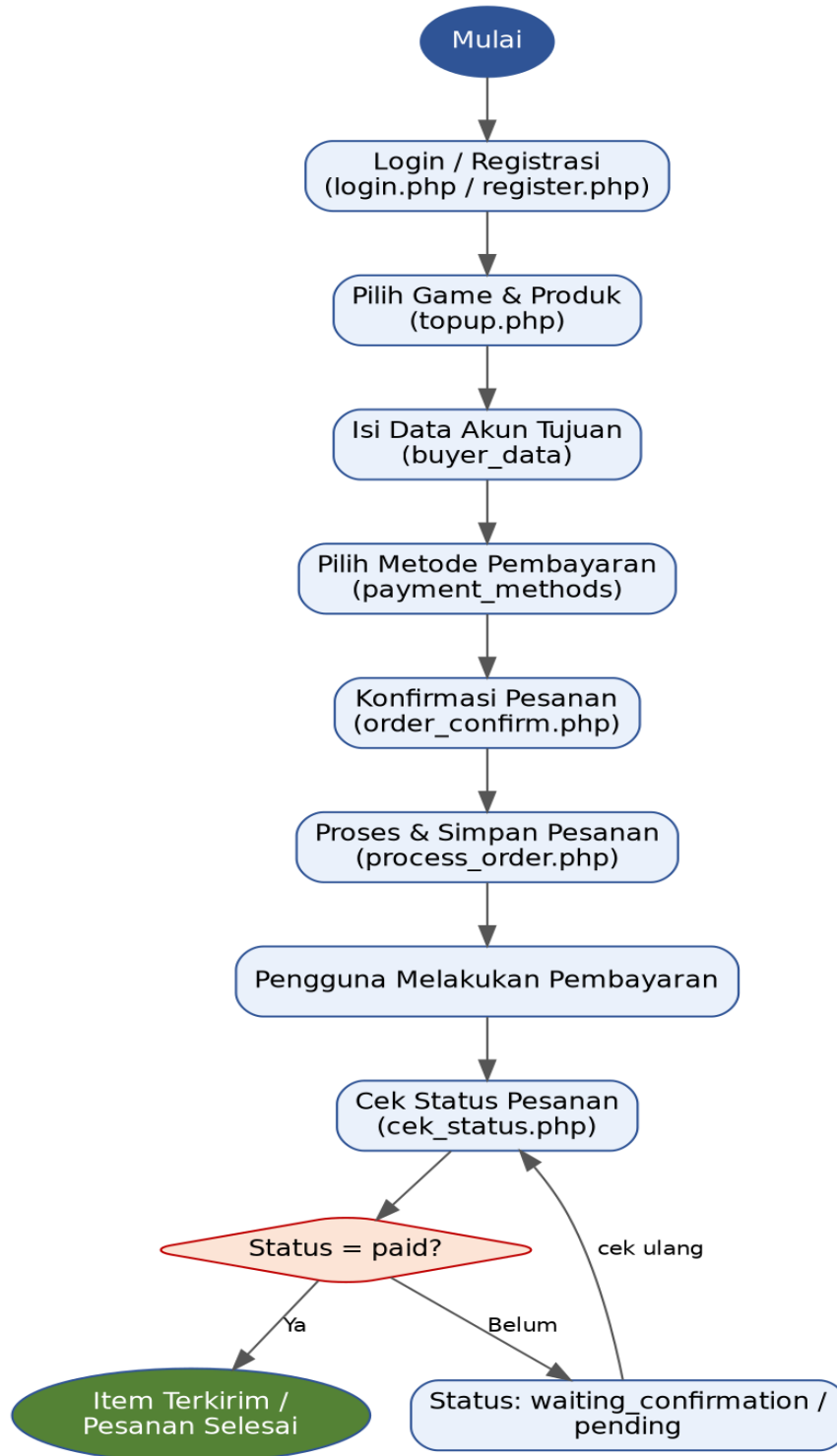
Gambar 3.2 Flowchart alur pemesanan top up
